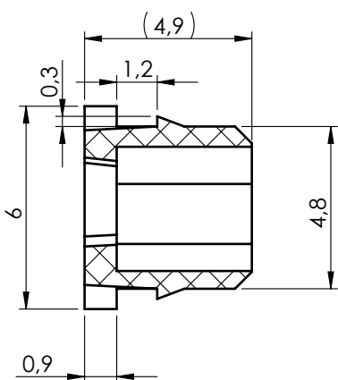
SECTION B-B SCALE 5 : 1
