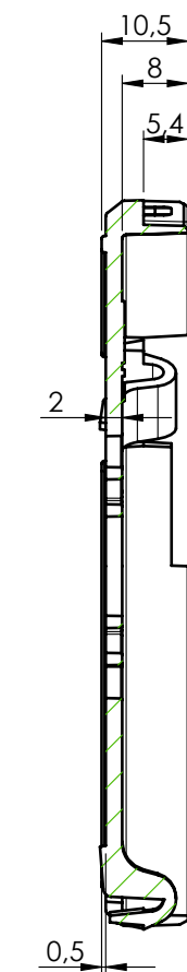
SECTION A-A
