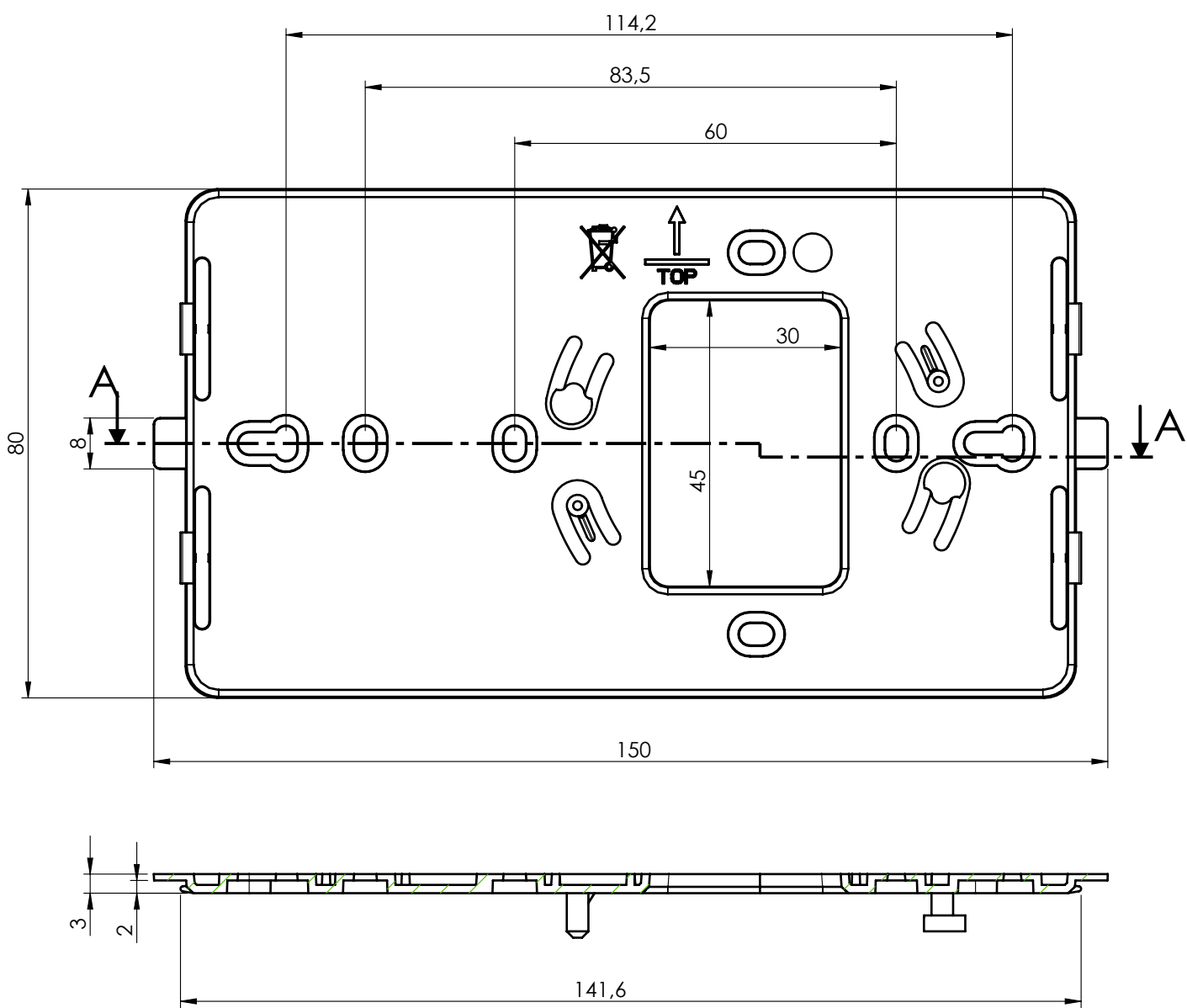
SECTION A-A
